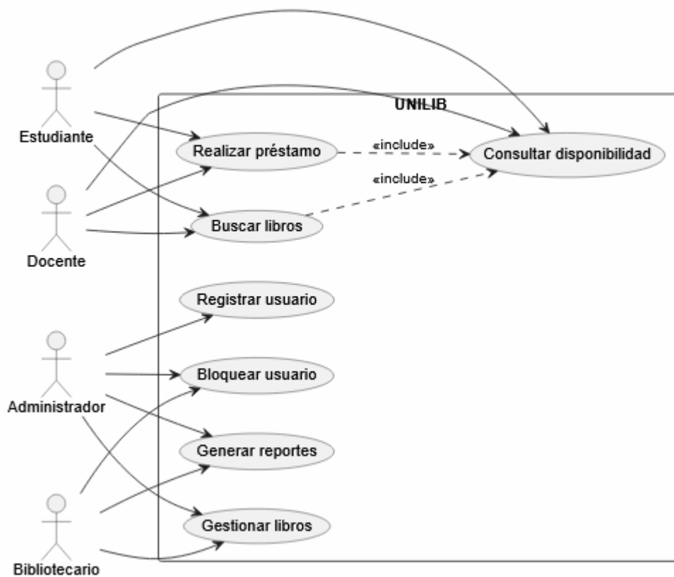
UNILIB - Diagrama general de casos de uso
