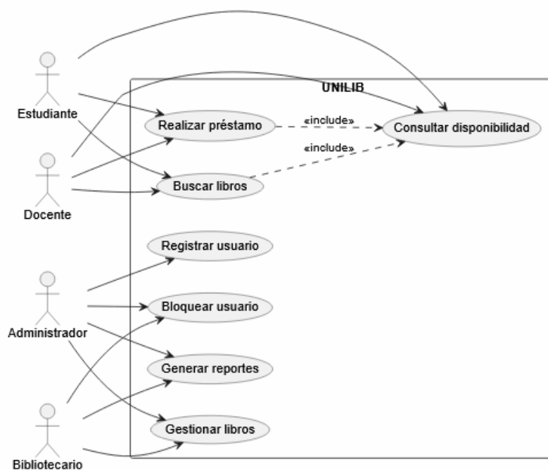
UNILIB - Diagrama general de casos de uso
